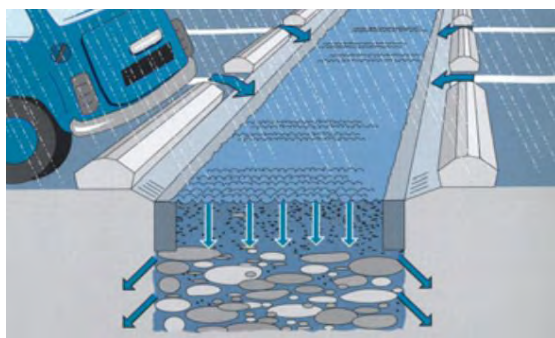
Figure 46 : Exemples de tranchées d'infiltration (Région Rhône-Alpes, 1994)
