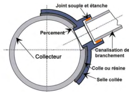
Figure 74: Exemple de selle collée
