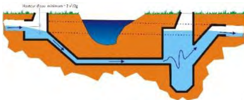
Figure 121 : Fonctionnement d'un siphon ; le siphon « tire ».
