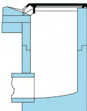
Figure 78 : Dispositif d'engouffrement non sélectif à passage direct
