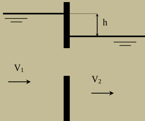
Vue en coupe d'un orifice noyé
