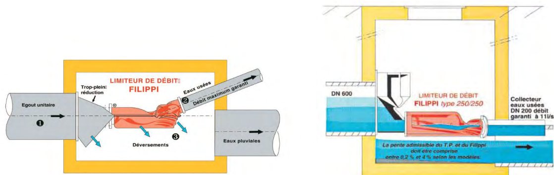
Figure 133 : Déversoir Filippi
