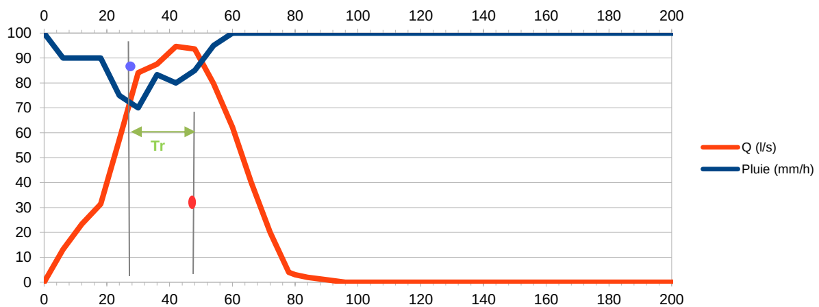
Figure 22 : Estimation graphique de t_r
