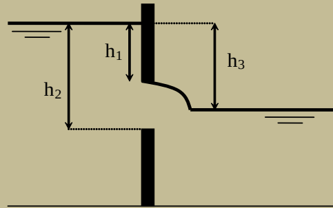
Vue en coupe d'un orifice partiellement noyé
