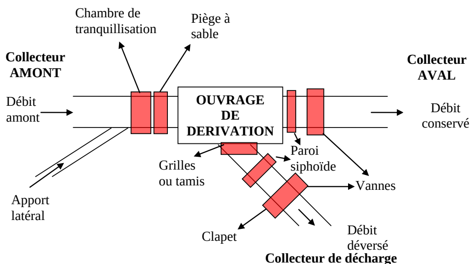
Figure 115 : Conception détaillée d'un déversoir d'orage
