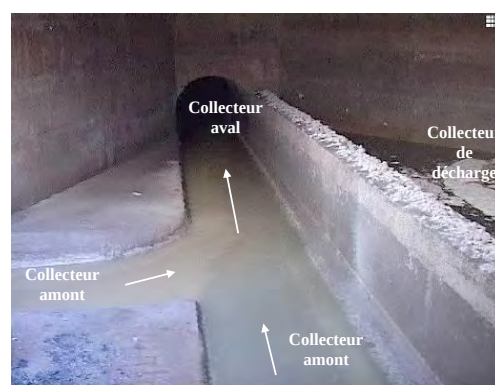
Déversoir complexe
