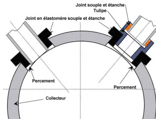
Figure 75 : Exemples de raccordement par joint en élastomère avec et sans tulipe
