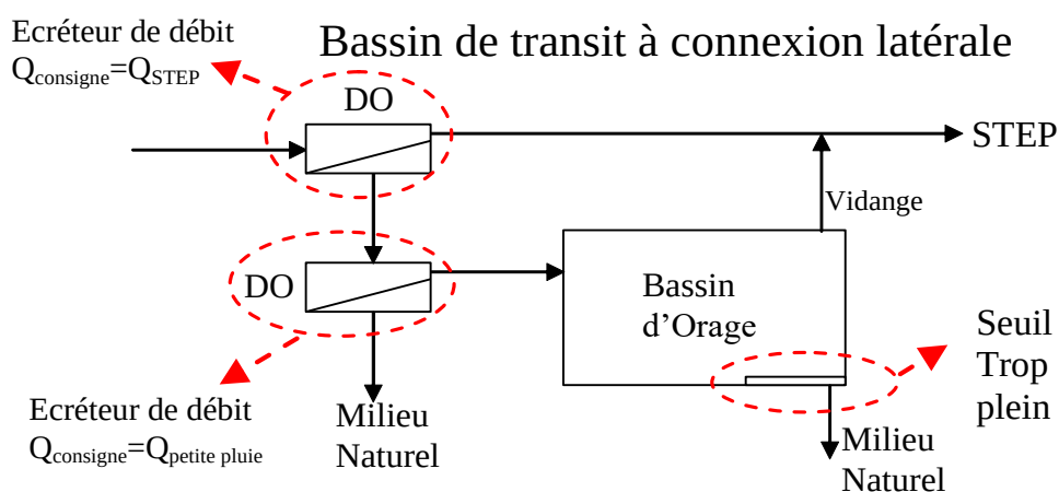
Figure 117 : Rôle des DO dans le fonctionnement d'un bassin de transit à connexion latérale
